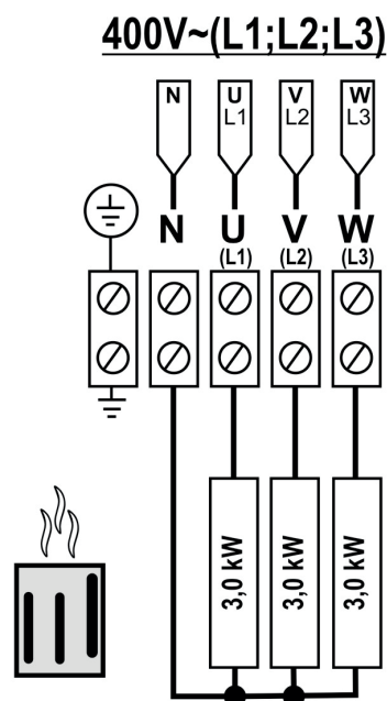
Externé riadenie saunovej pece 9 kW
